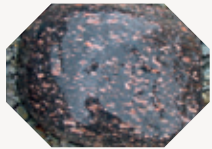
Granito e Gneis
